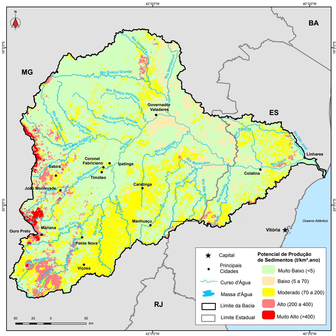
Figura 3. Potencial de produção de sedimentos na bacia, calculado em toneladas por quilômetro quadrado por ano
