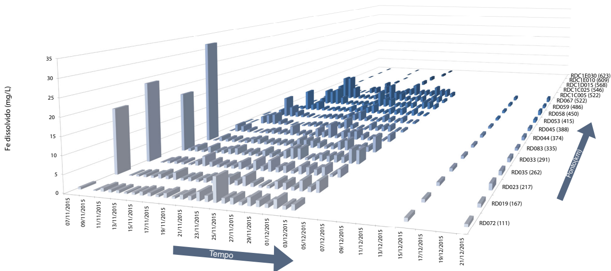
Figura 22. Ferro dissolvido no rio Doce após o rompimento da barragem Fonte: Elaborado a partir de dados do IGAM e IEMA
