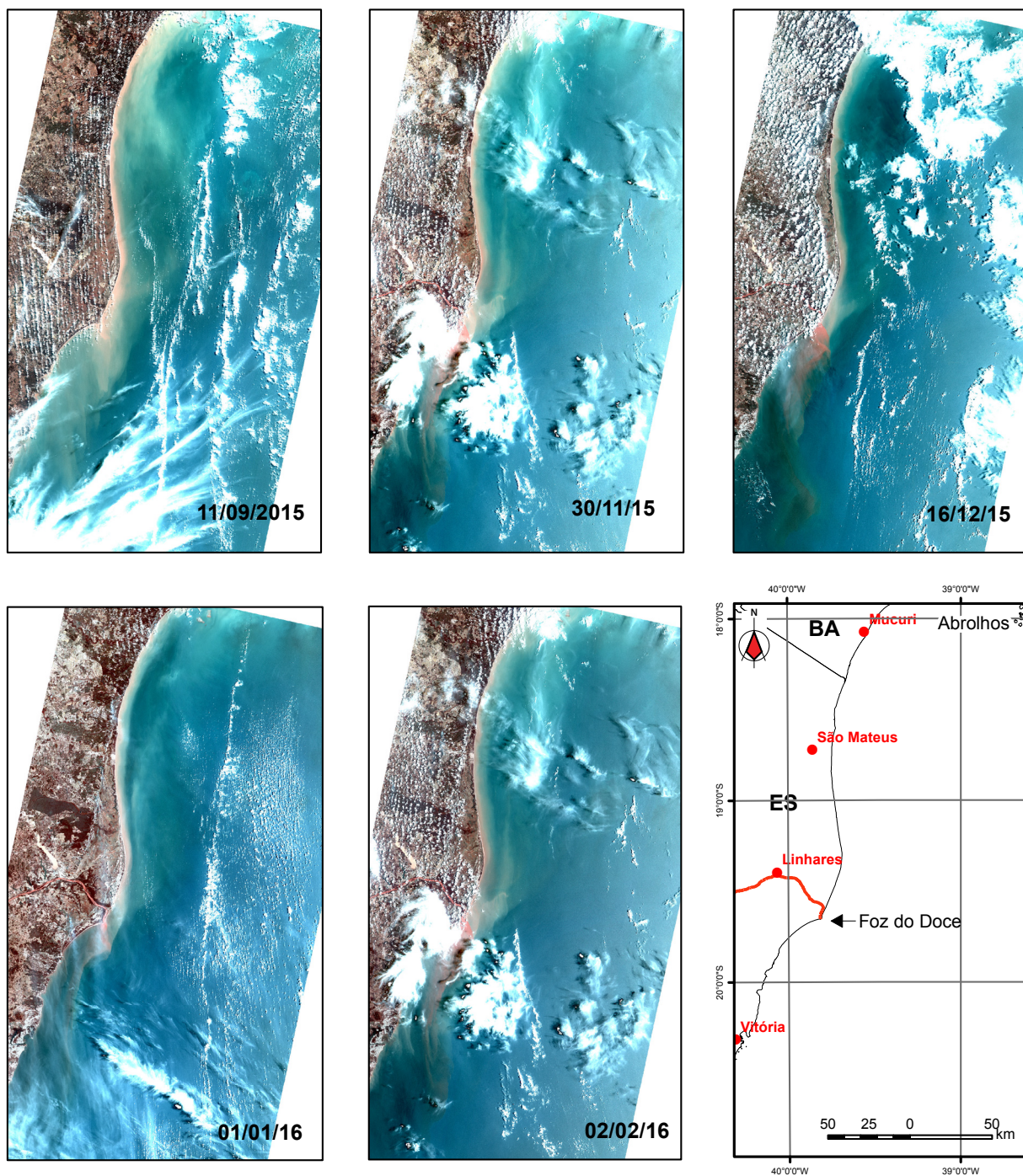
Figura 17. Série temporal de imagens do satélite Landsat 8 da região da foz do Doce Nota: Composição colorida de bandas R3G2B1. Fonte: Elaborado a partir de imagens do United States Geological Survey (USGS)
